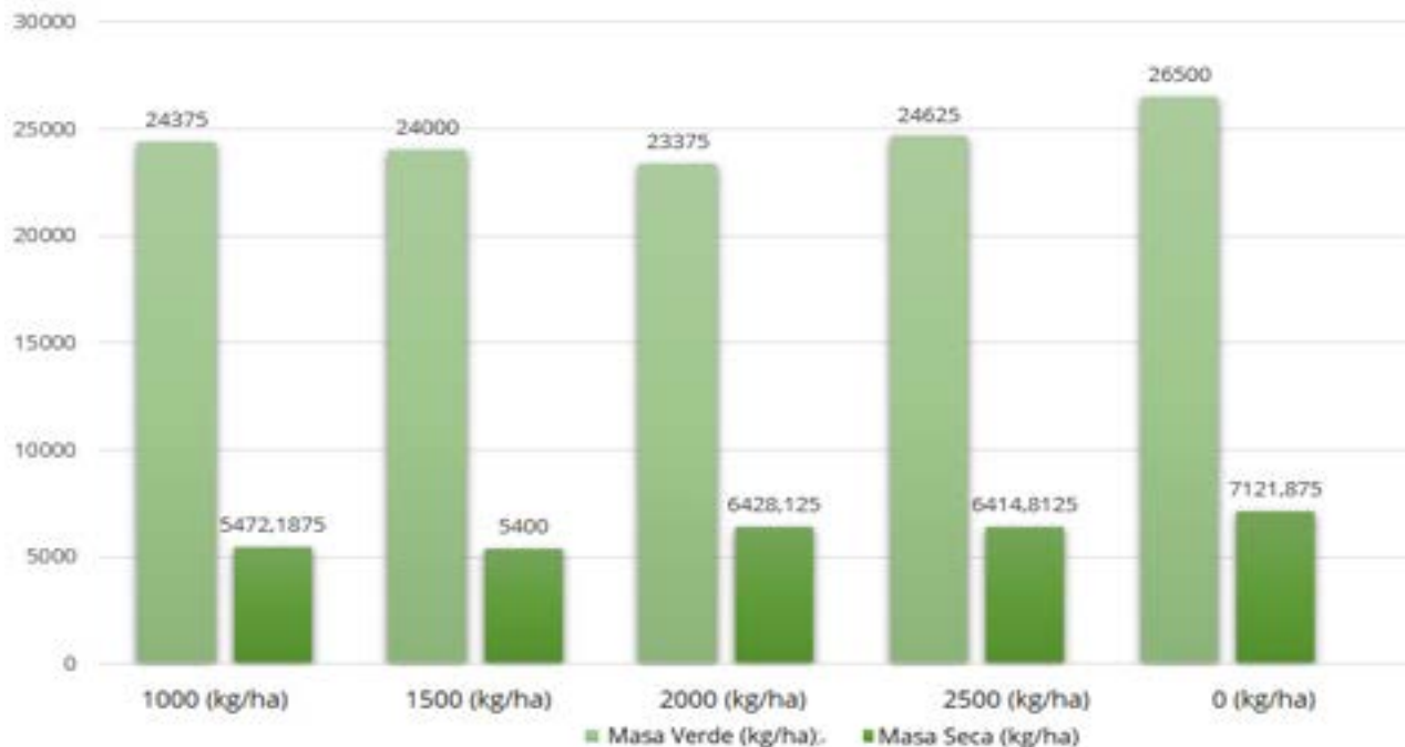
Figura 2.- Producción de biomasa húmeda y seca de pasto Urochloa brizantha ( Brachiaria brizantha cv. Marandú) en suelos de tierra firme con diferentes enmiendas de cal dolomita.
