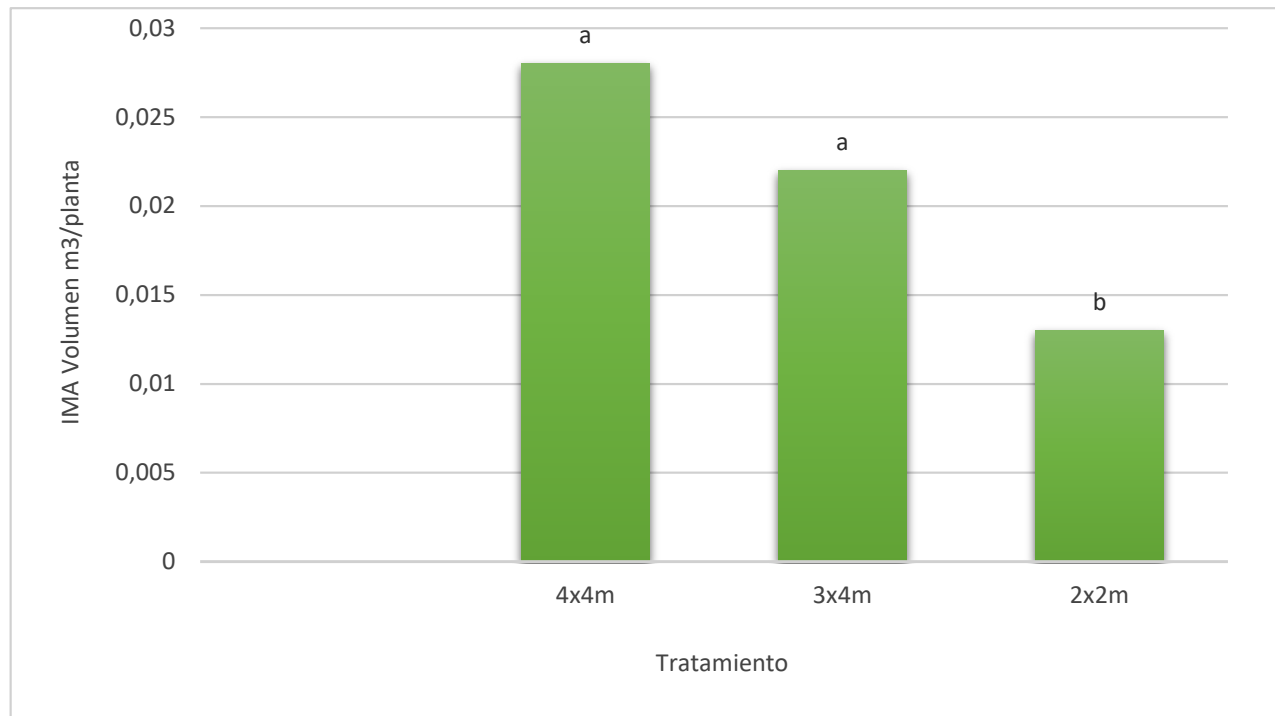
Figura 1. Incremento medio anual del volumen individual (m 3 ) de plantas de Balsa sembradas en diferentes espaciamientos.
