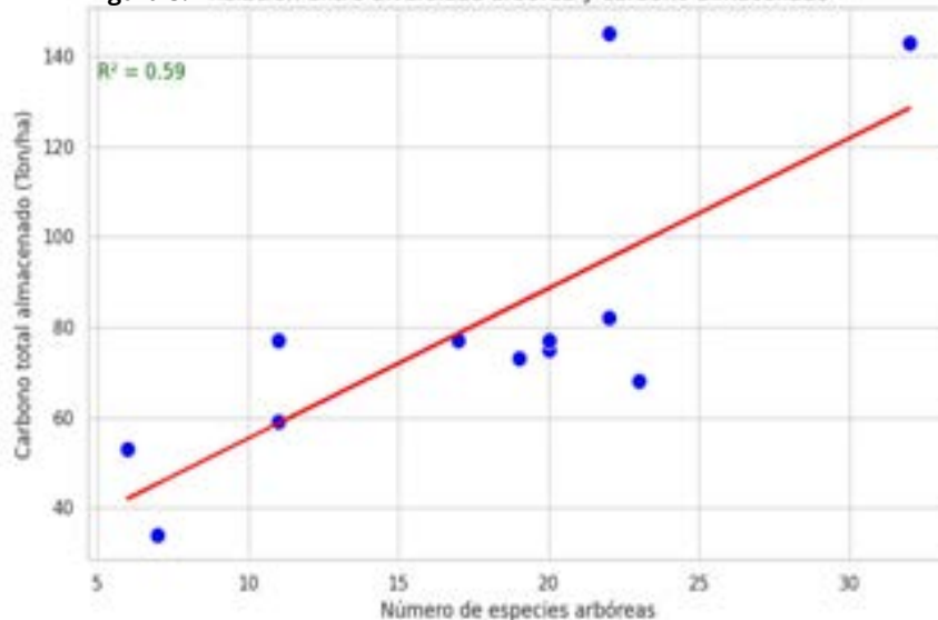
Figura 3.- Relación entre diversidad arbórea y carbono almacenado
